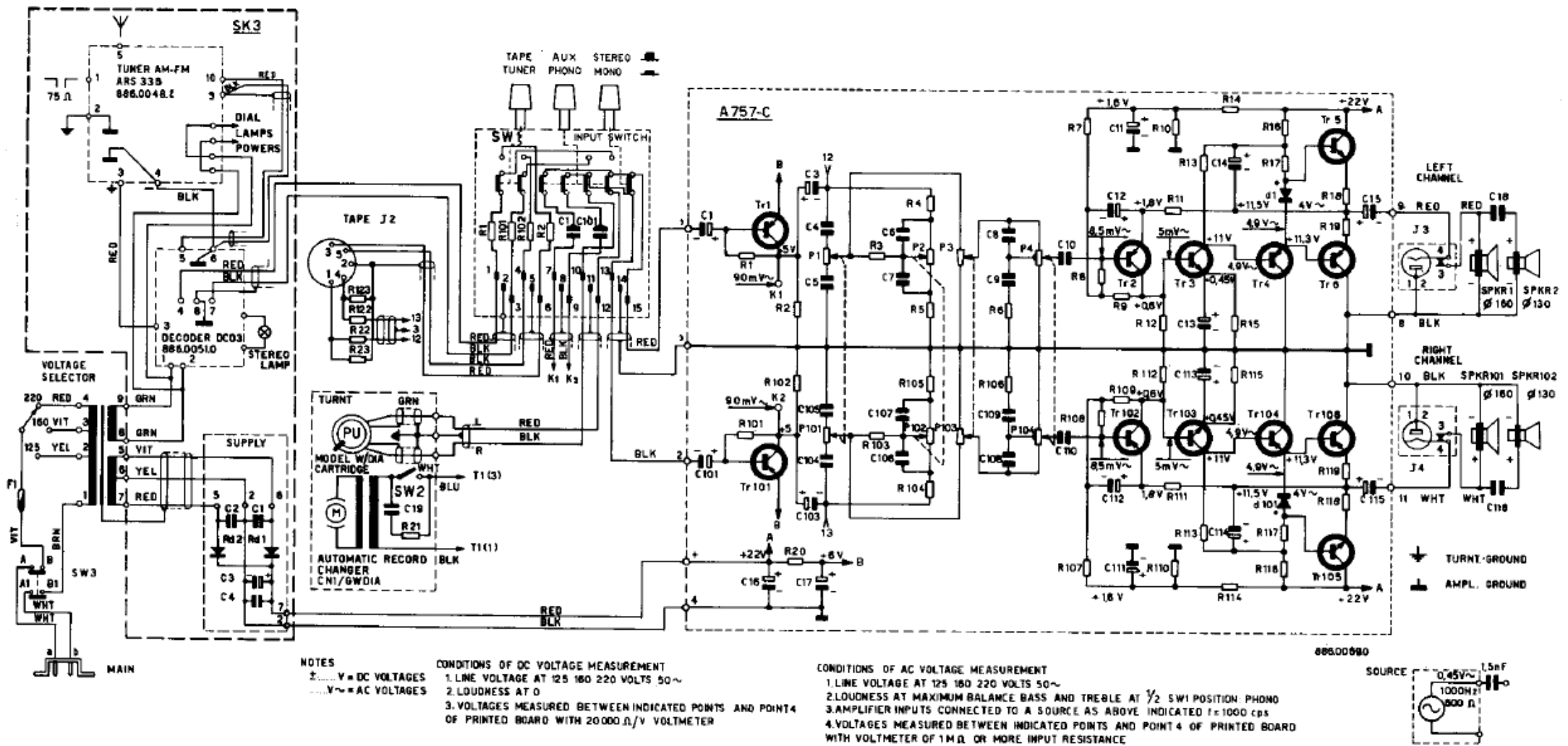
Fig. 12 — Schema elettrico LF 758/R
